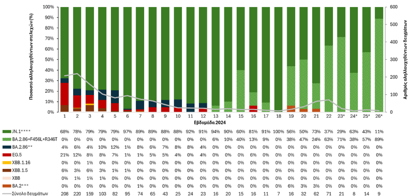
Διάγραμμα 16. Ποσοστό αλληλουχθέντων δειγμάτων ανά παραλλαγή επιδημιολογικού ενδιαφέροντος, ανά εβδομάδα, έως 28/06/2024
