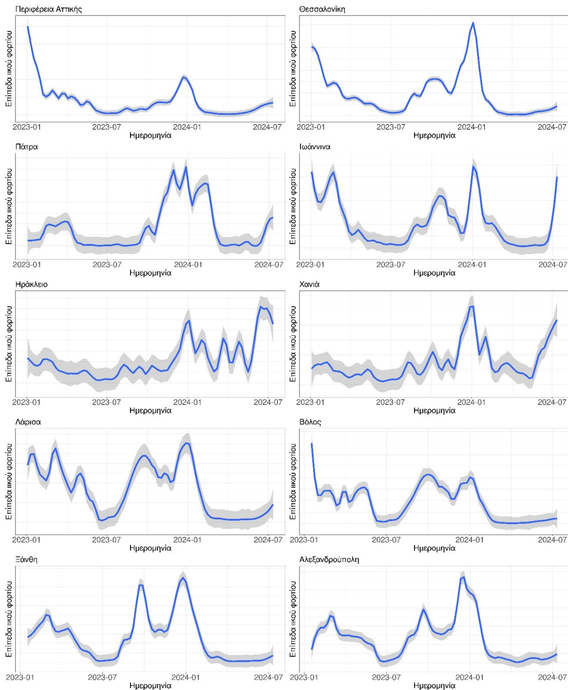
Διάγραμμα 18: Διακύμανση επιπέδων ιικού φορτίου (γονιδιακά αντίγραφα/100.000 πληθυσμό) στα αστικά λύματα συναρτήσει του χρόνου κατά την περίοδο 01/01/2023-14/07/2024
